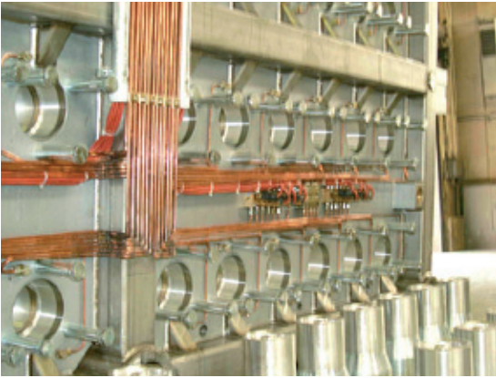
Übersicht Gießeinheit 48 x 4" Overview casting unit 48 x 4"
