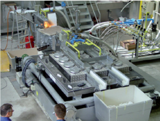
Übersicht Gießmaschine Overview castingmachine
